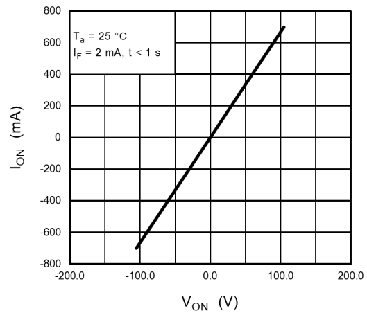
Fig. 12.1.4 I_{ON} - V_{ON}
