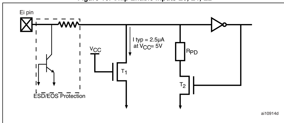
Figure 16. Chip Enable inputs E0, E1, E2
