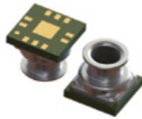
CCLGA 10L (3.3 x 3.3 x 2.9 mm)
