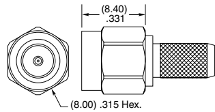
-ST-C10
