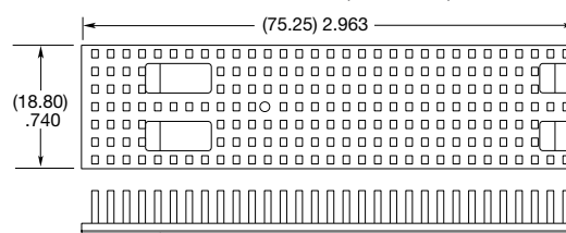
HS-QSFP-DD-P1-2 SHOWN
