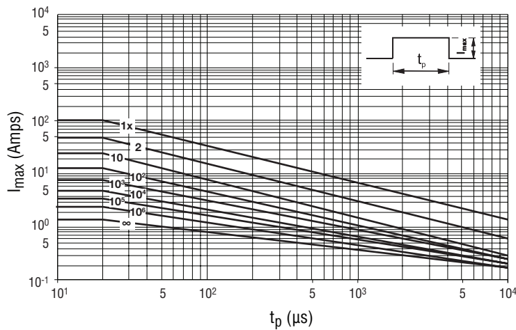
Model Size 0805 - (ZV 8 L 0805 121 HT ~ ZV 30 K 0805 121 HT)
