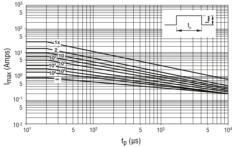
Model Size 0805 - (ZV 2 M 0805 101 HT ~ ZV 6 M 0805 101 HT)
